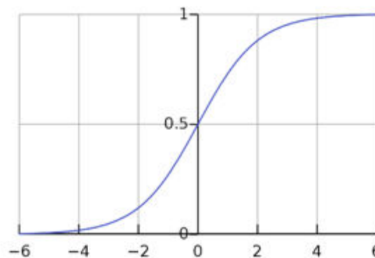
Fig.12. Sigmoid function chart.
